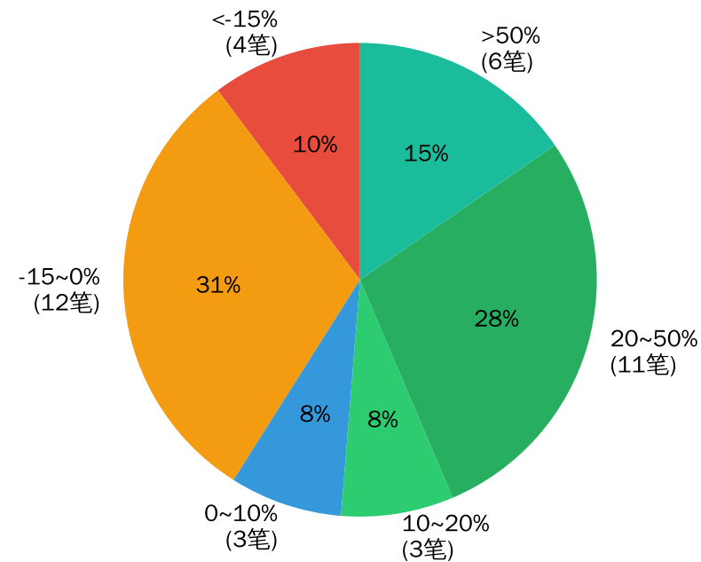
收益分布
